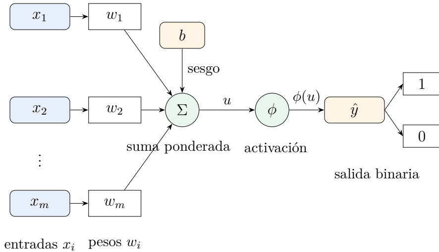
Figura 1: Diagrama del perceptrón: suma ponderada de las entradas y función de activación.
