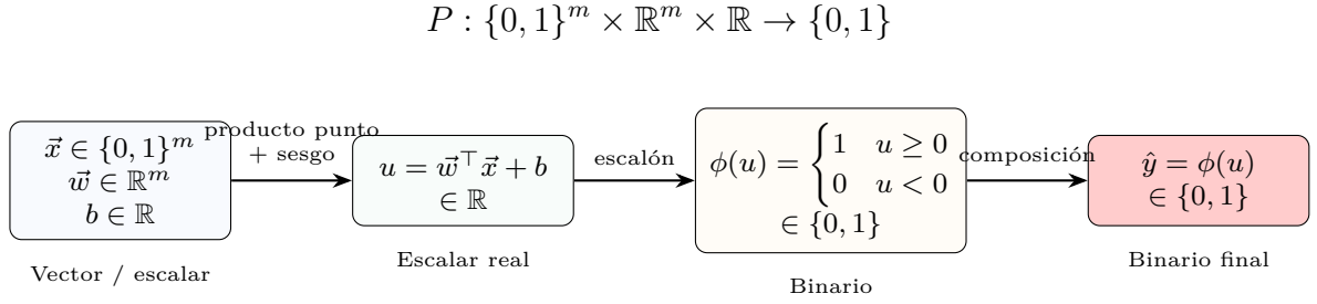
Figura 2: Recorrido de las variables en el perceptrón.
